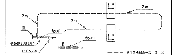
冷却水系統図
